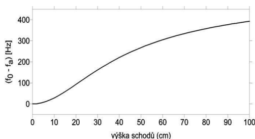
Obr. 17. Závislost f_0 - f_a na výšce schodu \Delta y pro typickou šířku schodu \Delta x = 30 cm
