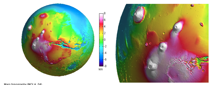
Mars topography (MOLA_04)
